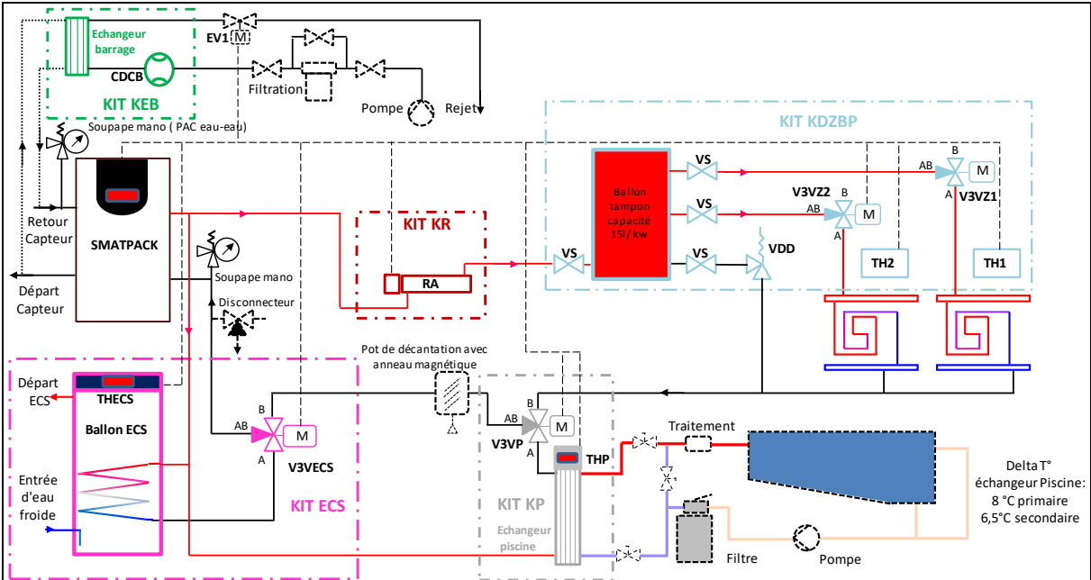
Schéma hydraulique générique d’une installation avec kit 2 zones plancher (kit KDZBP), ECS, résistance d’appoint, Piscine. ( à compléter suivant installation)
